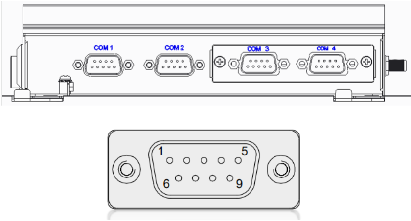
COM Port 1/Port 2 RS-232 (Default)
