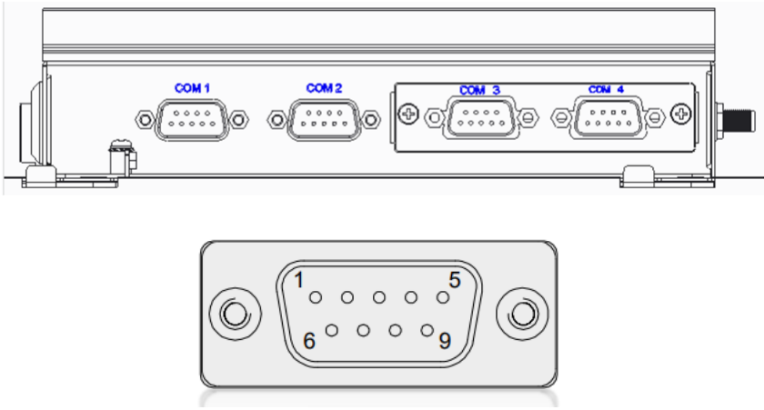
COM Port 3/Port 4 RS-232 (Default)
