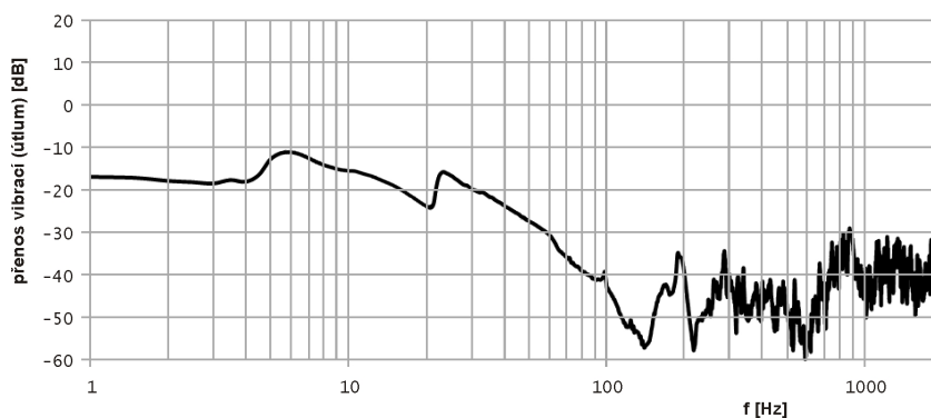
Graf útlumu vibrací 1 Hz ÷ 1 kHz
