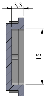
SEZIONE A-A
