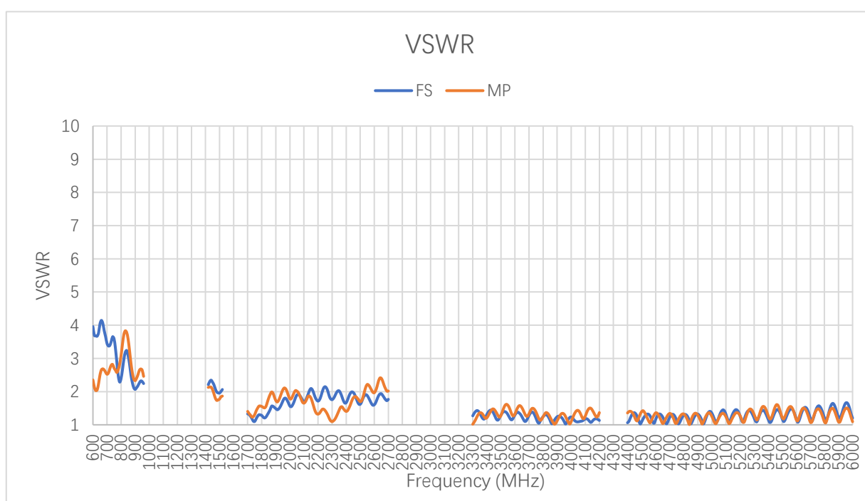
VSWR
