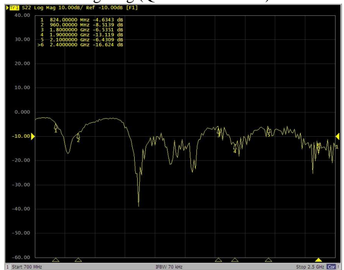
Log Mag (Quad Band + WiFi)
