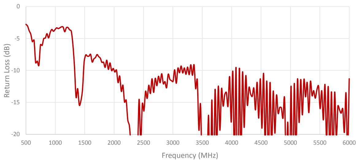
Cable 4: 5GNR
