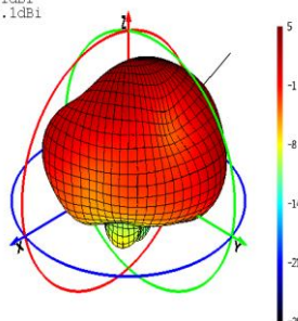
2450 MHz
