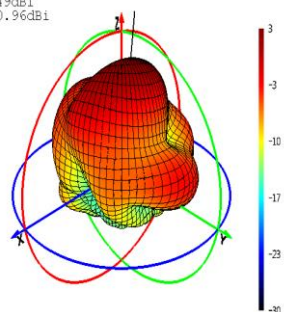
2450 MHz
