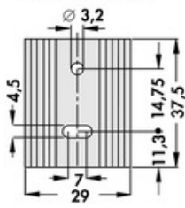
SK 09 37,5 TO 220
