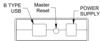
UNO/101 PANEL
