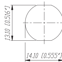
Frontplattenausschnitt (Rückseite) Panel cut out (rear side)
