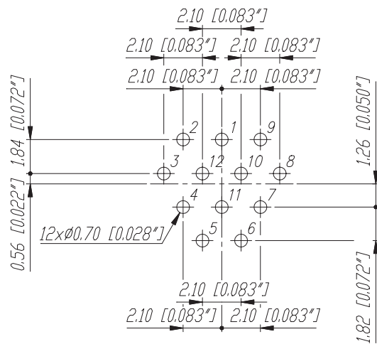
Print-Bohrplan (Bestückungsseite) PCB-Layout (component side)
