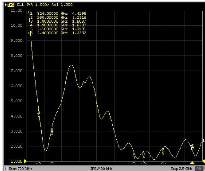
VSWR
