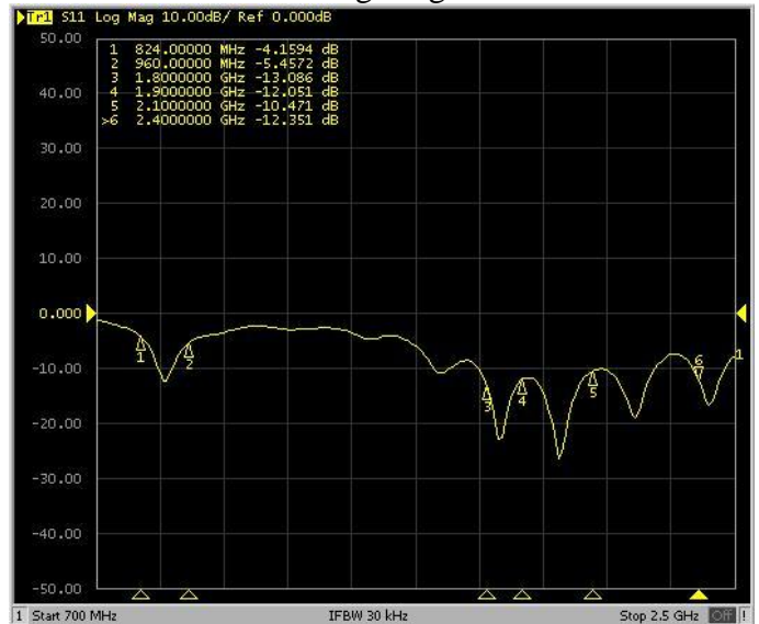
Log Mag
