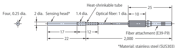
E32-T222, E32-T222R
