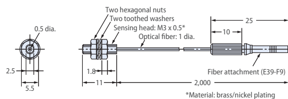
E32-TC200F, E32-TC200FR
