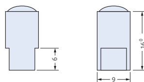
E39-EF51
