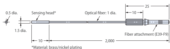
E32-T223R
