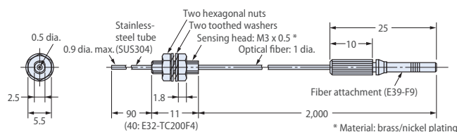
E39-EF1-37
