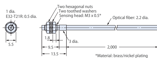
E32-TC200B, E32-TC200BR
