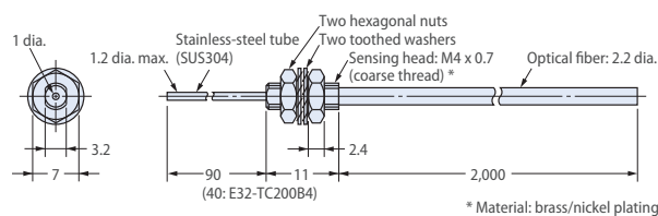
E32-TC200E
