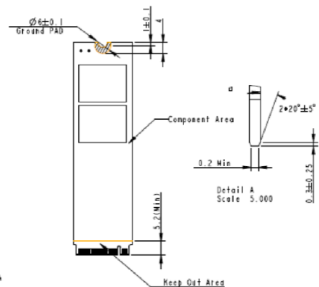
Bottom side
