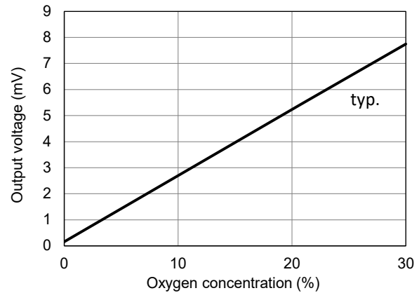
Fig. 3b - KE-50LF sensitivity characteristics
