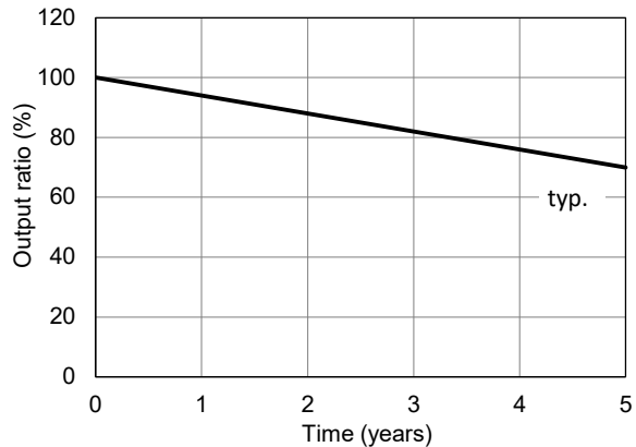
Fig. 9a - KE-25LF long term stability
