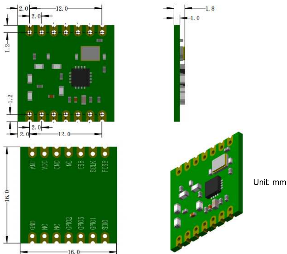
Figure3. Dimensions
